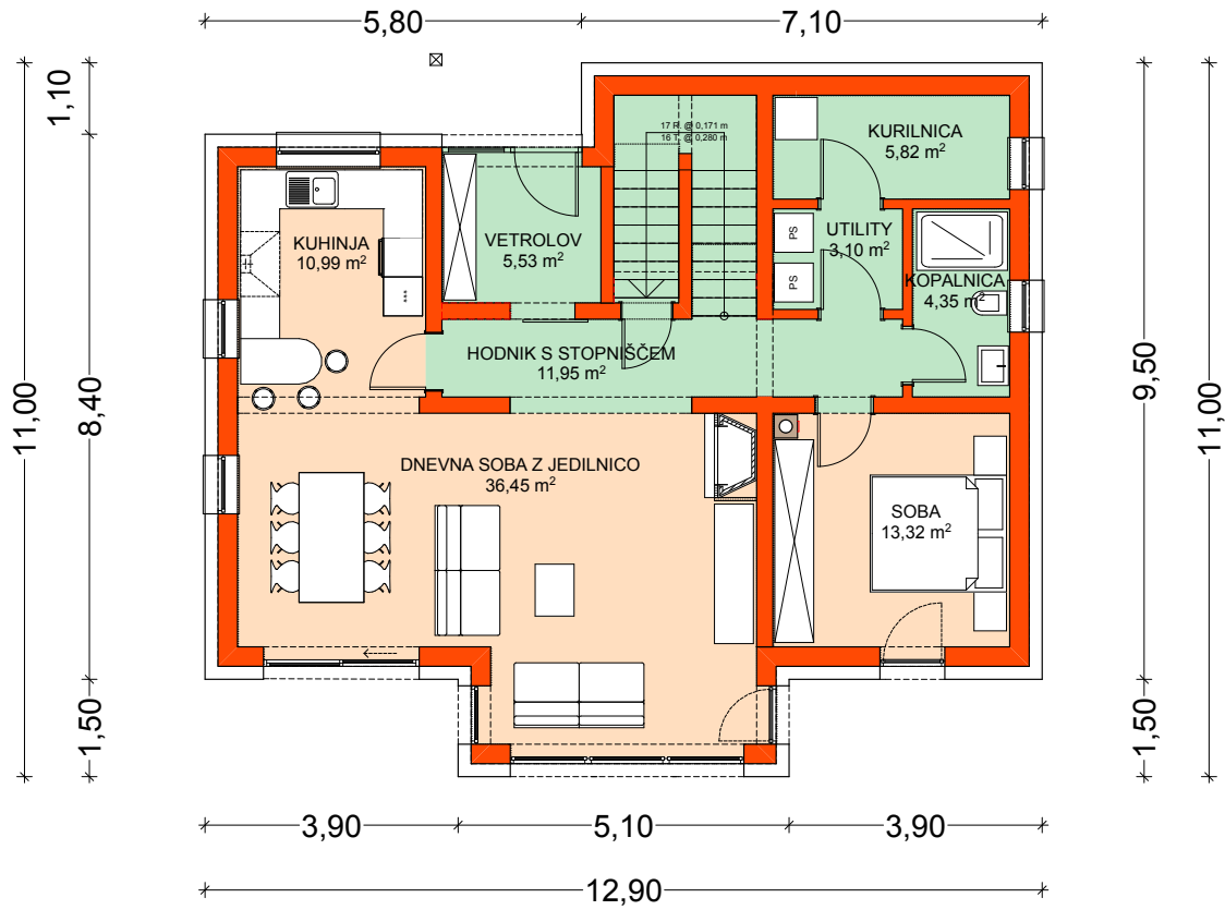
PRITLIČJE skupna površina: 91,51 m 2
